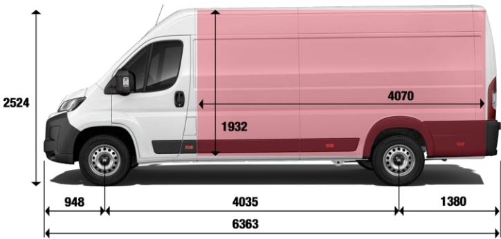
FURGON - L4H3 - 17 M 3
