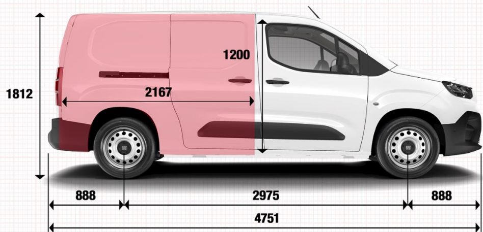
CREWCAB L2 - 1,8 M 3 / 3,5 M 3 / 4,0 M 3 *
