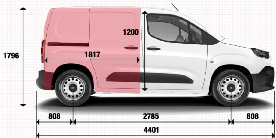
FURGON L2 - 3,9 M 3 / 4,4 M 3 *
