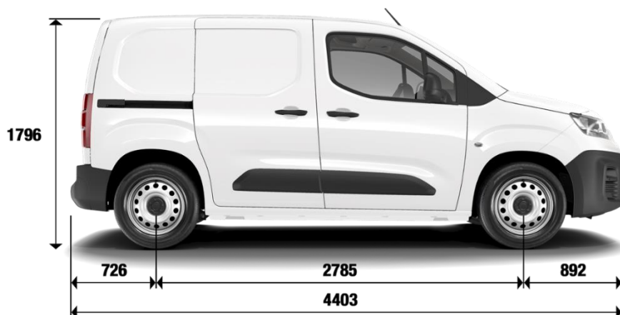
FURGON L1 - 3,3 M 3 / 3,8 M 3 *
