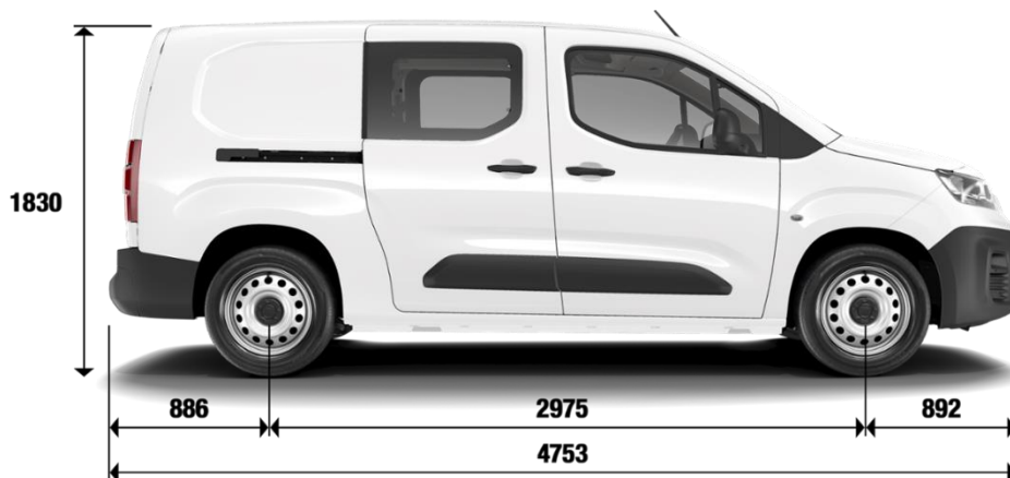
CREWCAB L2 - 1,8 M 3 / 3,5 M 3 / 4,0 M 3 *
