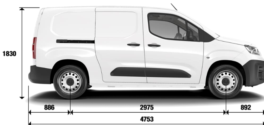
FURGON L2 - 3,9 M 3 / 4,4 M 3 *
