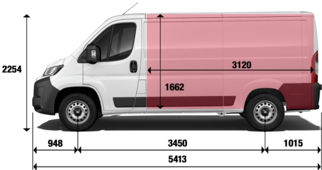
FURGON - L2H2 - 11,5 M 3
