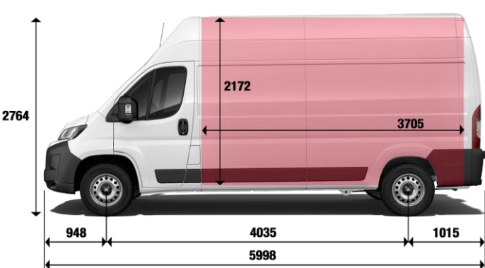
FURGON - L3H3 - 15 M 3
