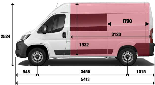
FURGON - DUPLA KABINA, 7 SEDEŽEV - L3H2 - 10,5 M 3
