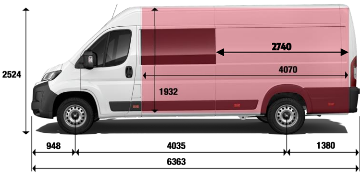
FURGON - DUPLA KABINA, 7 SEDEŽEV - L4H2 - 12,5 M 3
