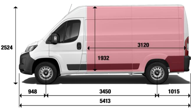
FURGON - L3H2 - 13 M 3
